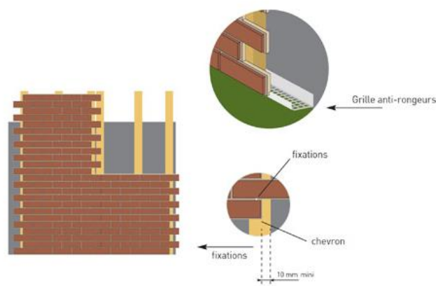
Principe de montage VETAblic (bardage) sur béton ou maçonnerie
